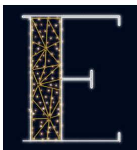
LETTRE E MAJ OR 204803-24V H 1,7 x W 1,31 m. 10 Kg. 29 W.
