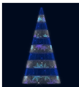
SAPIN FLOCONS XL BLEU 204782-24V H 10 x W 5 x D 5 m. 401 Kg. 1084 W.
